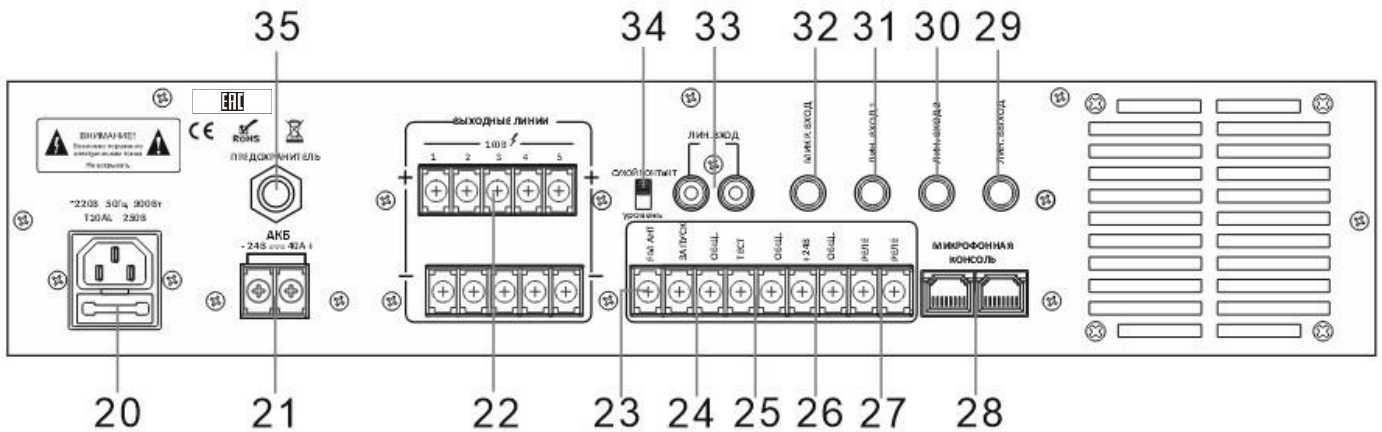
Рис. 1.3. Задняя панель
