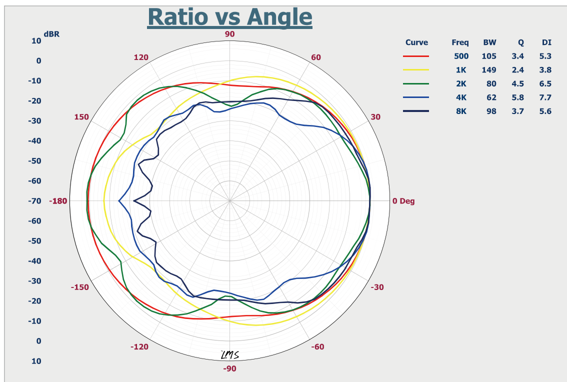
Круговая диграмма направленности громкоговорителя LPA-10N
