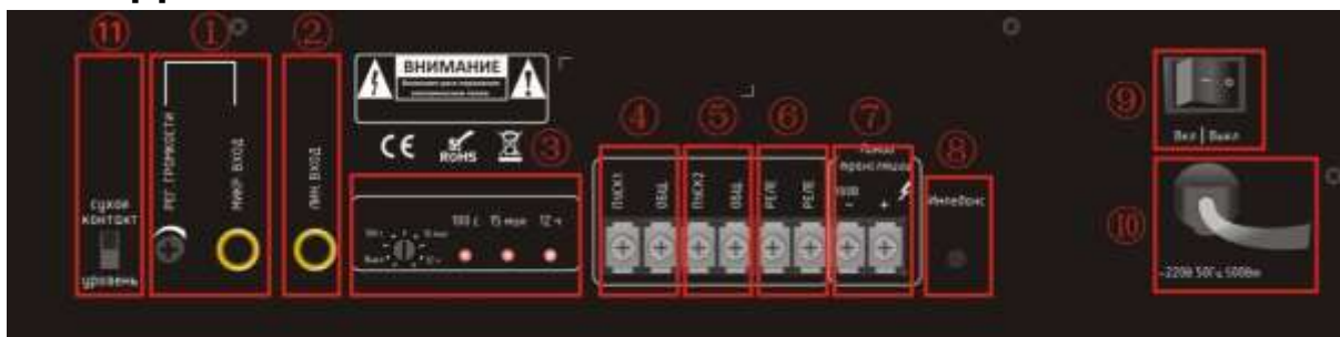
Рис. 1.3. Задняя панель LPA-MINI300
