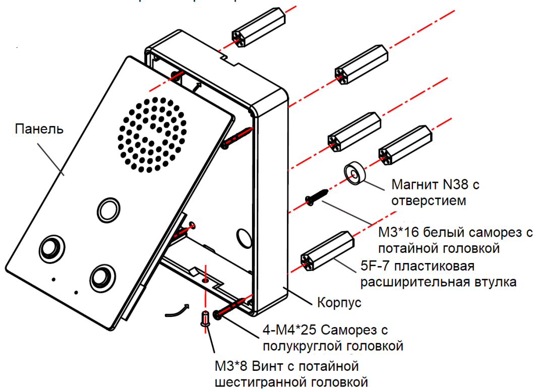
Схема установки Габаритные размеры в мм
