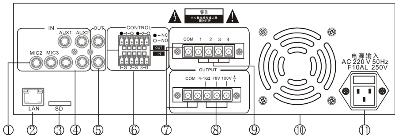
Рис.2.2. LPA-2301NBSP06
