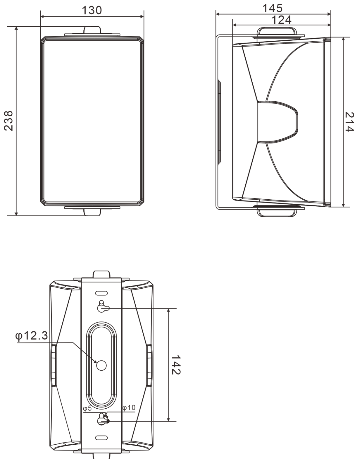
Рис 4. Настенный IP-громкоговоритель LPA-6013GEN
