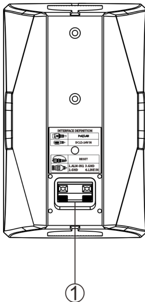
Рис. 3. Задняя панель настенного IP-громкоговорителя LPA-6013GEN
