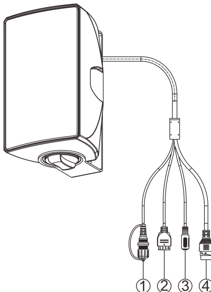
Рис. 2. Интерфейсы настенного IP-громкоговорителя LPA-6013GEN
