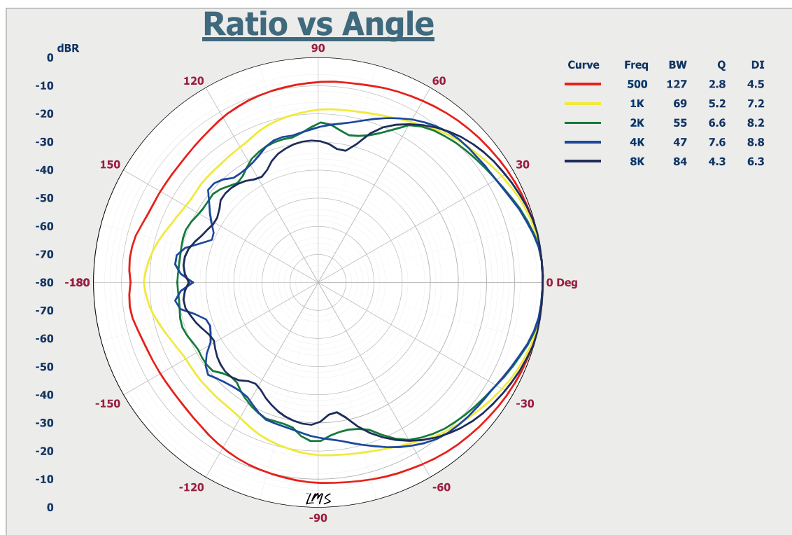
Круговая диаграмма направленности громкоговорителя LPA-300H12
