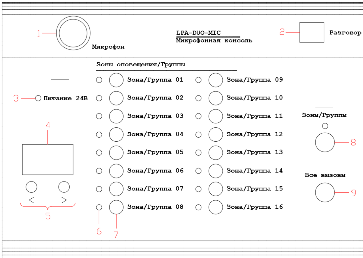
Рис. 2.1. LPA-DUO-MIC (передняя панель)
