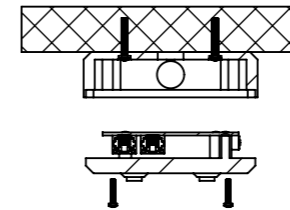
B-B (1 : 5)
