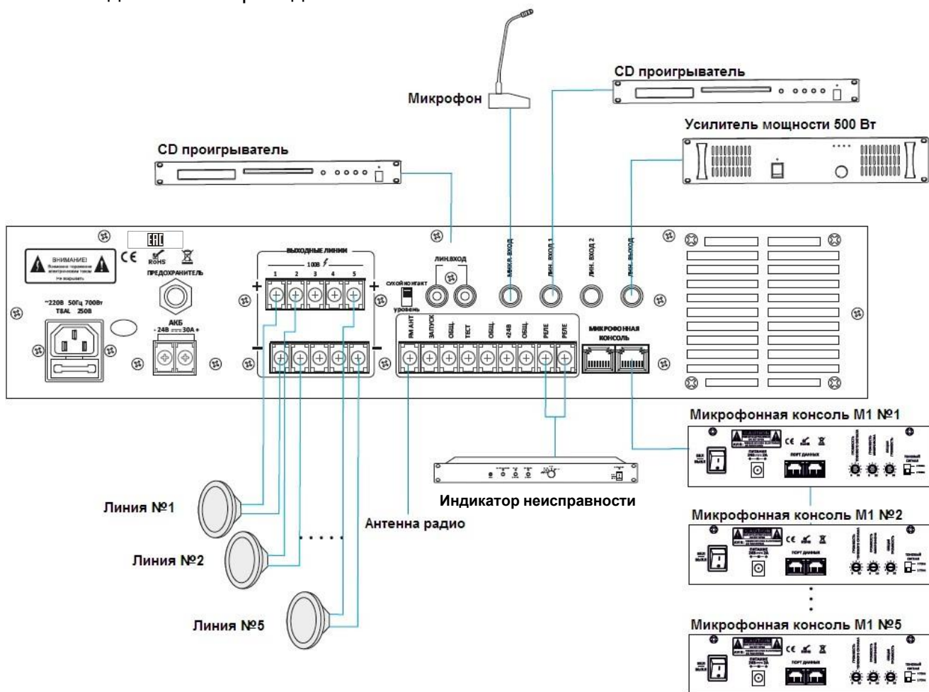
Рис. 2.1. Схема подключения
