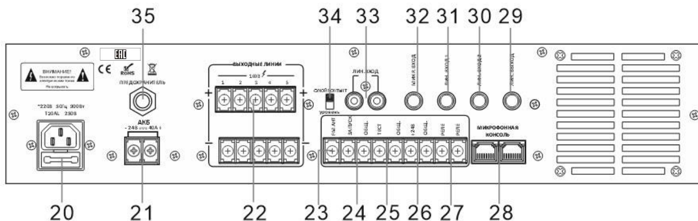
Рис. 1.3. Задняя панель
