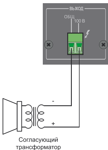
Рис. 2.2. Схема подключения громкоговорителей к LPA-TA-35M
