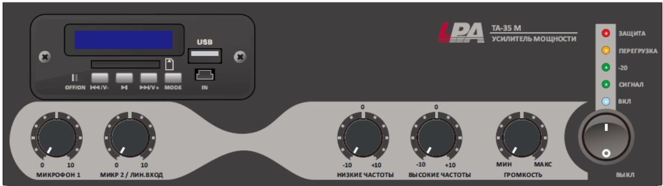
Рис. 1.1. LPA-TA-35M
