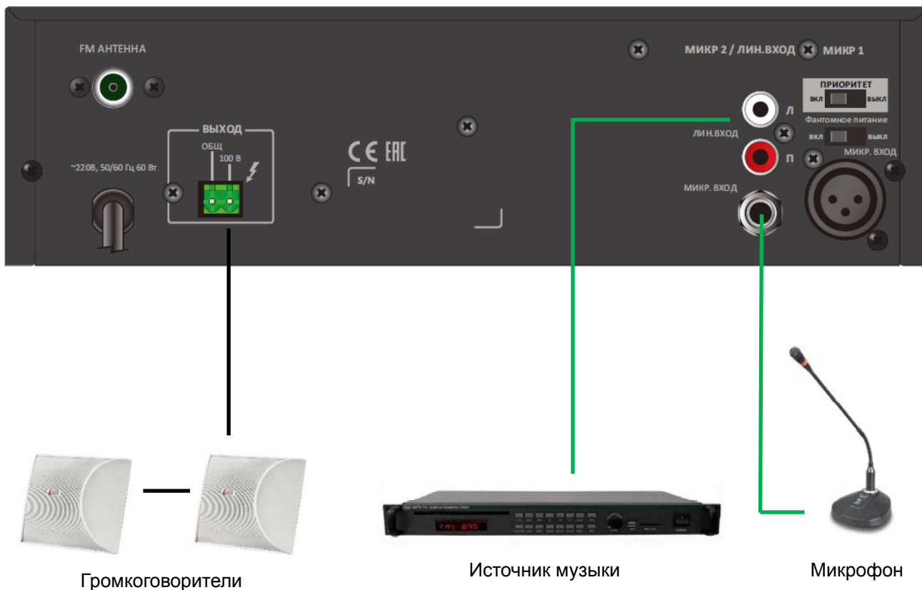
Рис. 2.1. Схема подключения LPA-TA-35M
