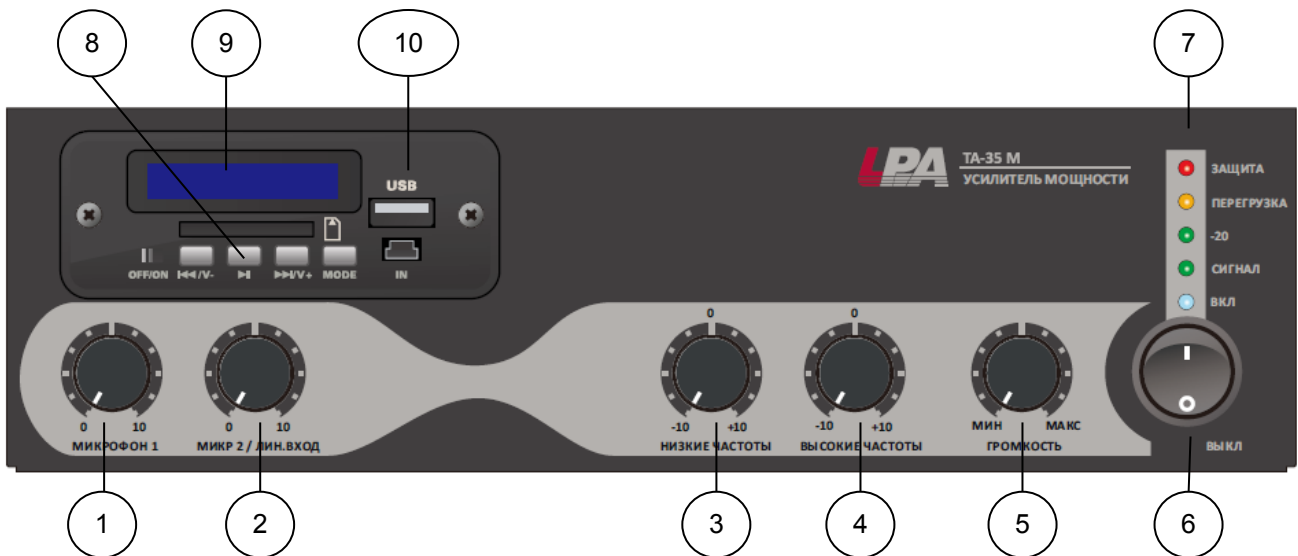
Рис. 3.1. Схема расположения средств управления LPA-TA-35M
