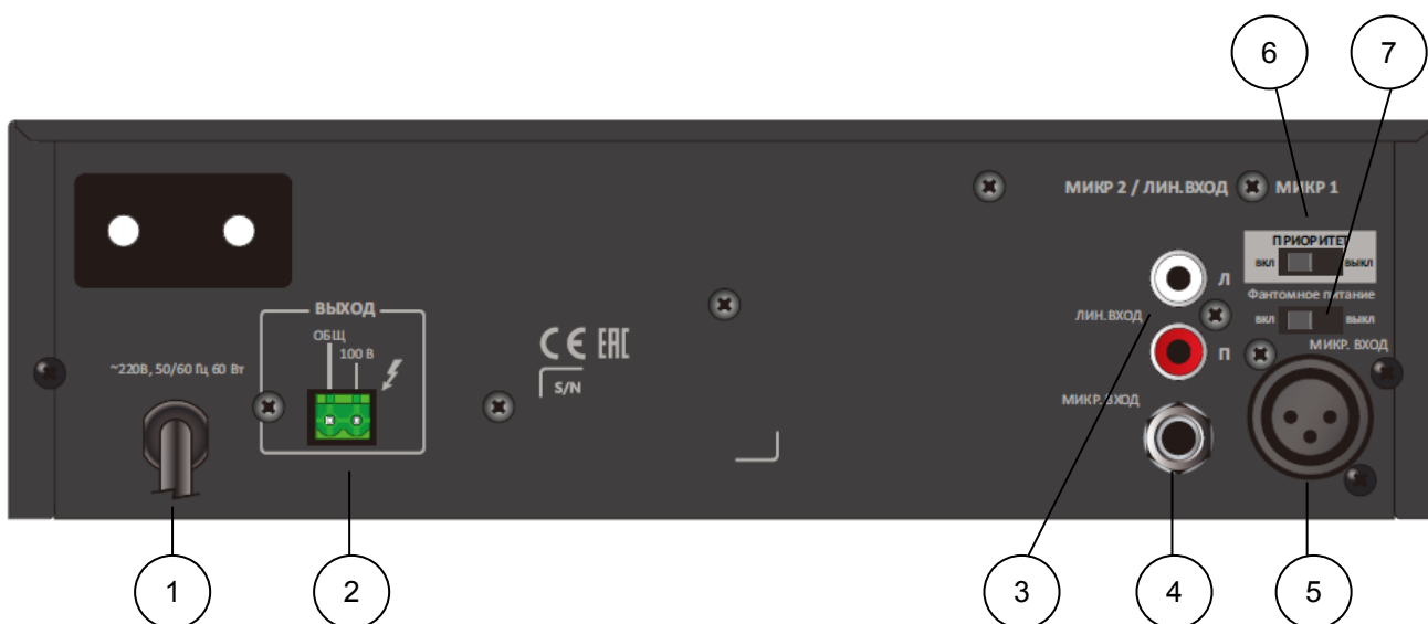
Рис. 3.2. Схема расположения средств управления LPA-TA-35M
