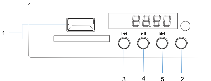
Рис. 3.10. Встроенный MP3 проигрыватель контроллера LPA-PRESTA-2.
