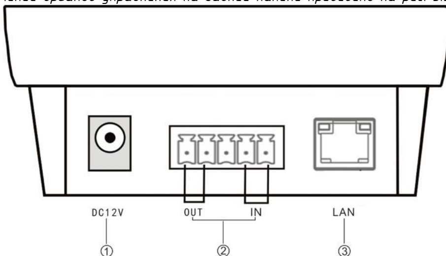
Рис.3.2. Задняя панель LPA-8526NAS
