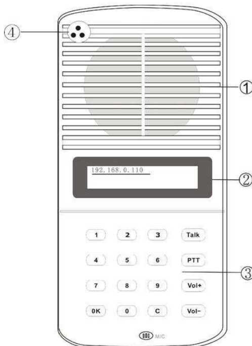
Рис.3.1. Передняя панель LPA-8526NAS
