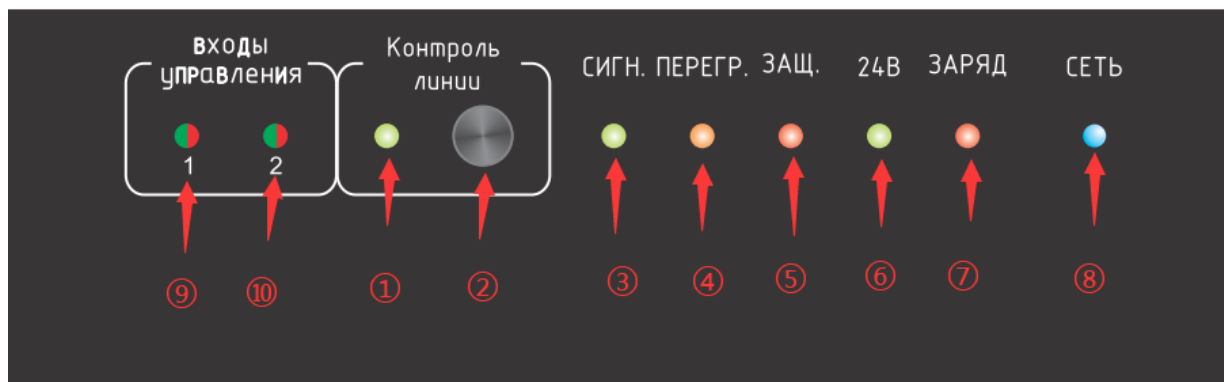
Рис. 1.2. Передняя панель
