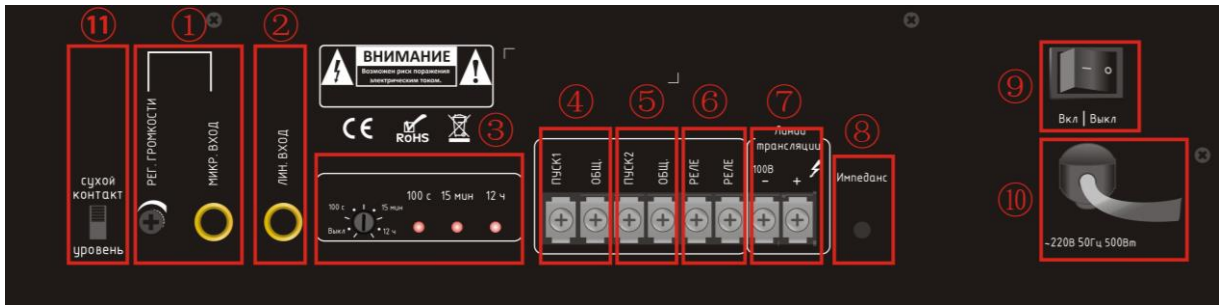
Рис. 1.3. Задняя панель
