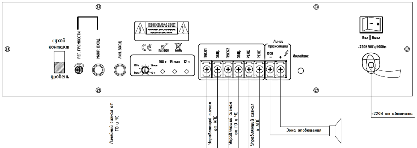
Рис. 2.1. Схема подключения
