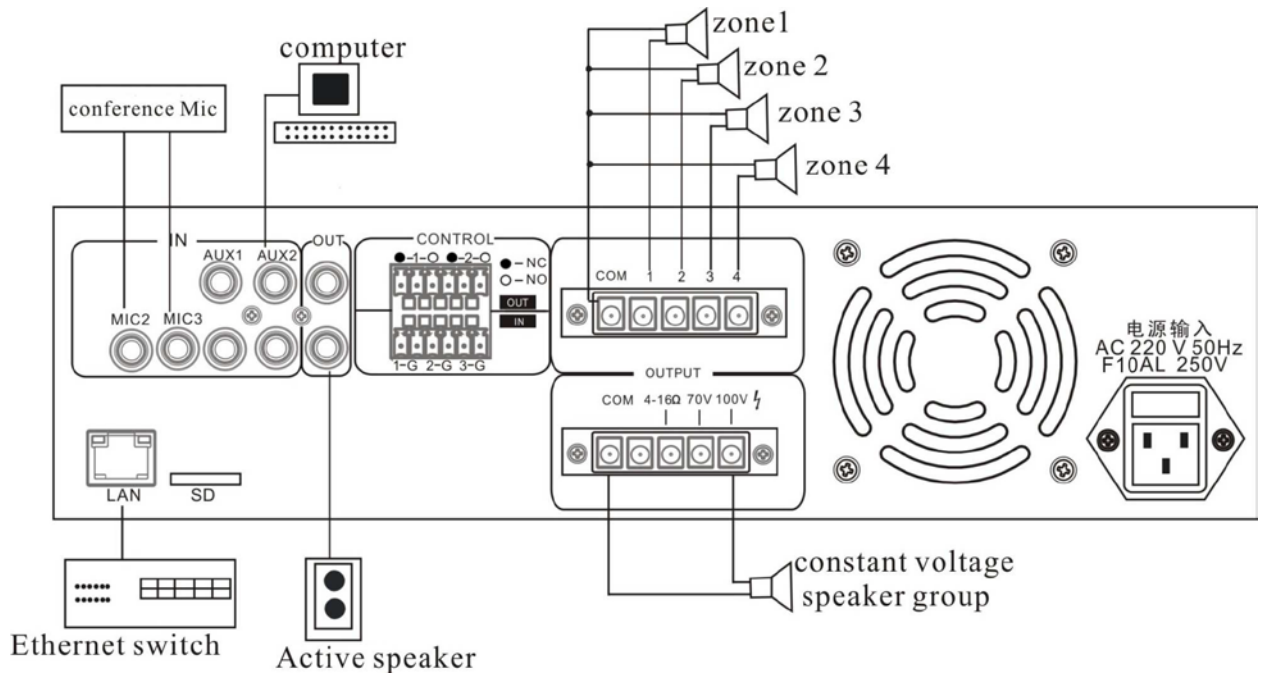
Рис.3.1. Схема подключения LPA-2301NBSP12
