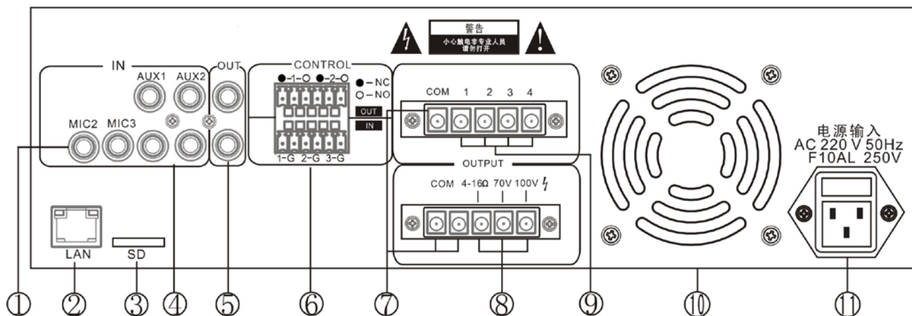
Рис.2.2. LPA-2301NBSP12
