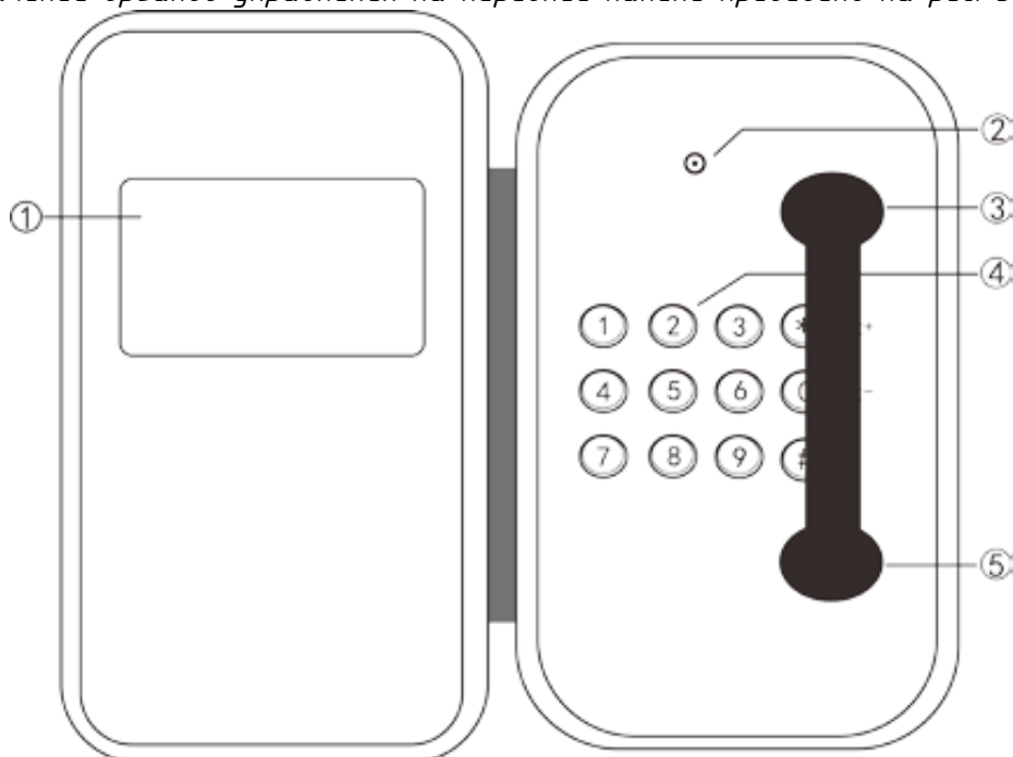
Рис.3.1. Передняя панель LPA-8519NAS
