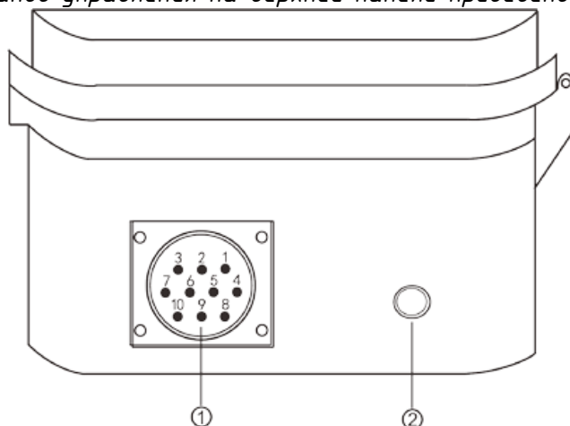
Рис.3.2. Верхняя панель LPA-8519NAS
